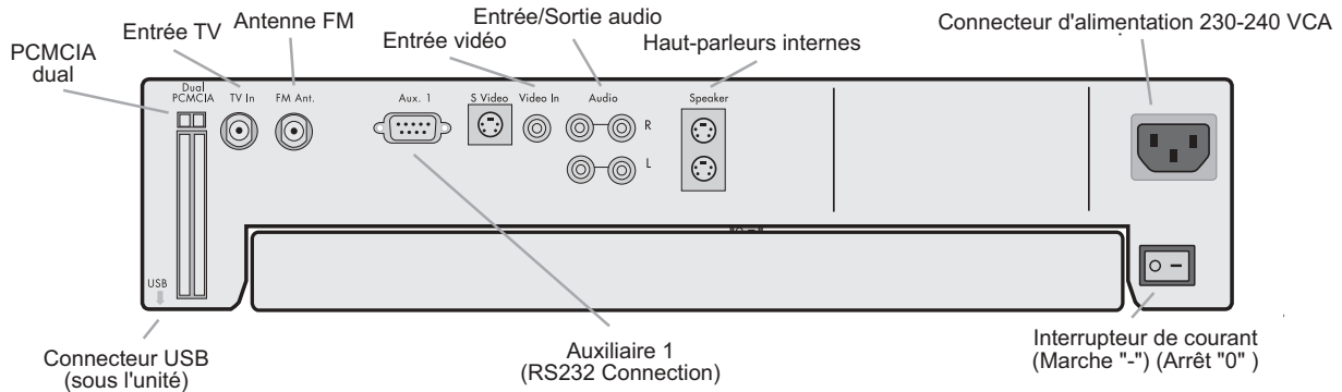
ILLUSTRATION 4. Panneau arrière de l'iCEBOX FlipScreen
