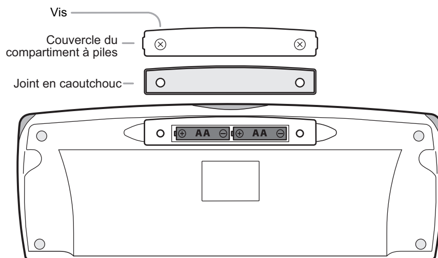
ILLUSTRATION 3. Installation des piles dans le clavier
