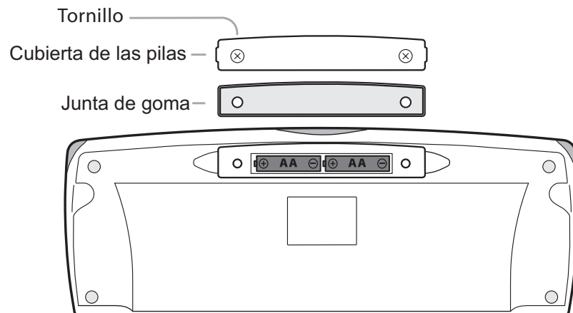
ILUSTRACIÓN 3. Instalación de las pilas del teclado
