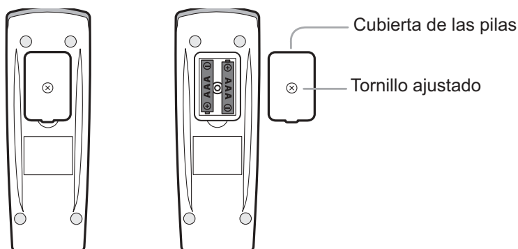
ILUSTRACIÓN 2. Instalación de las pilas del control remoto
