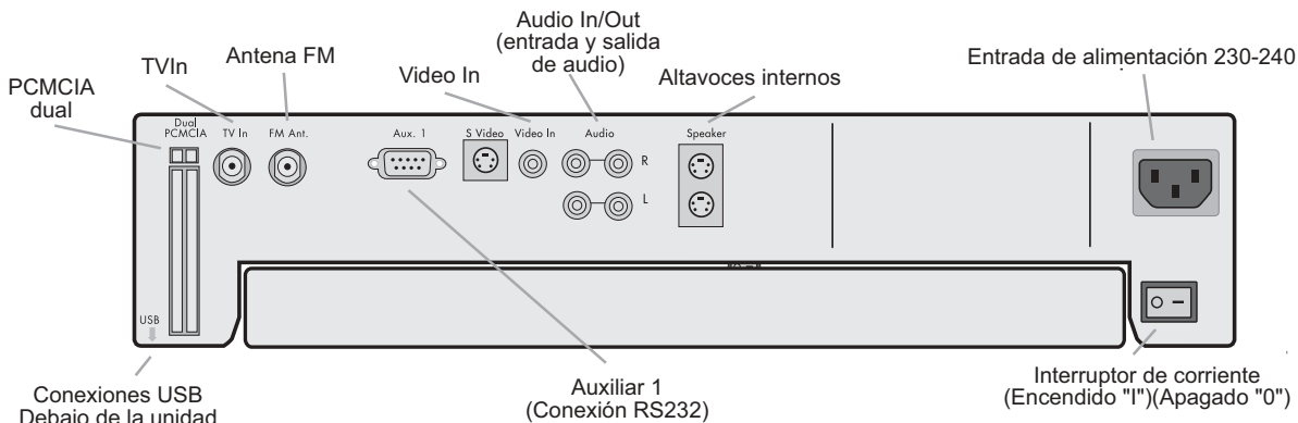
ILUSTRACIÓN 4. Panel trasero de la iCEBOX FlipScreen
